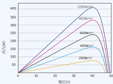
PVモジュール (410W) の P-V 曲線
